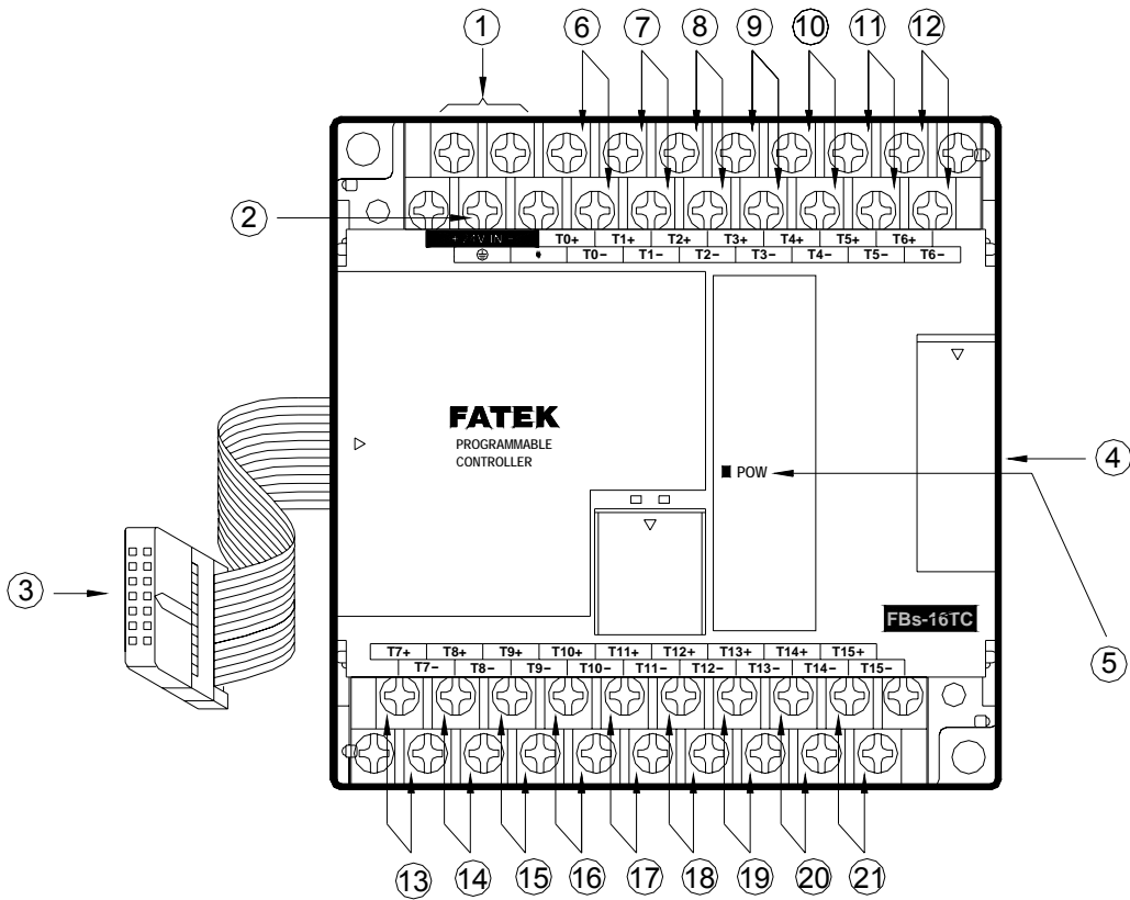
16TC 外觀正視圖
